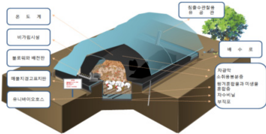
그림 3. 호기성호열미생물을 이용한 가축사체 처리 표준매몰지 부분 단면도
